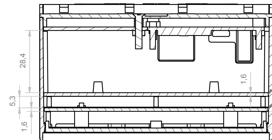
A-A (1:1)
